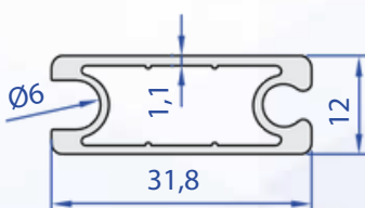
60107-00 0,334 kg/m
