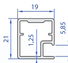
60211-00 0,300 Kg/m
