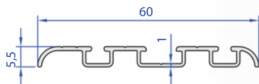
60390-00 0,270 Kg/m
