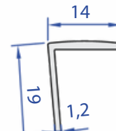
60020-00 0,113 kg/m
