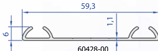
60428-00 0,254 Kg/m
