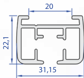
05074-00 0,545 kg/m
