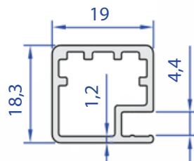
60394-00 0,280 Kg/m
