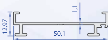
60104-00 0,292 kg/m
