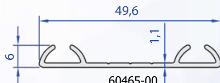
60465-00 0,225 Kg/m
