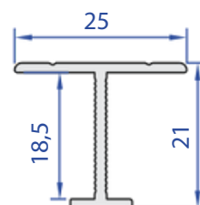
60363-00 0,191 Kg/m
