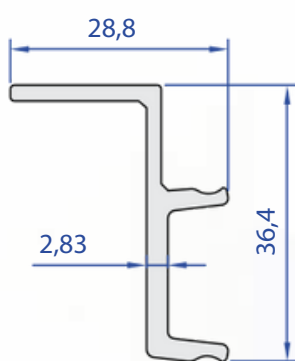
60572-00 0,438 Kg/m
