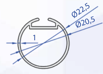
60040-00 0,212 kg/m
