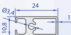
60087-00 0,253 kg/m
