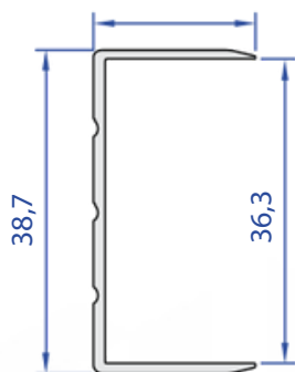
60466-00 0,251 Kg/m
