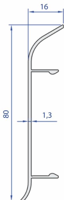
05715-00 0,391 Kg/m
