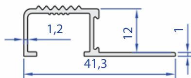
60086-00 0,236 kg/m
