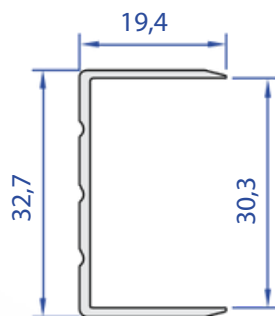
60413-00 0,228 Kg/m
