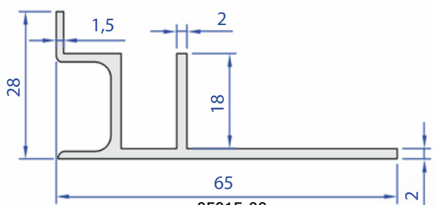
05015-00 0,616 kg/m
