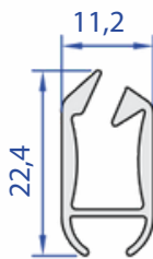
60127-00 0,222 kg/m
