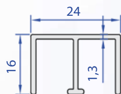
60136-00 0,250 kg/m
