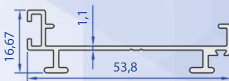
60149-00 0,337 Kg/m
