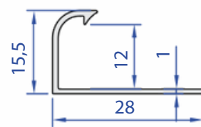
60072-00 0,132 kg/m
