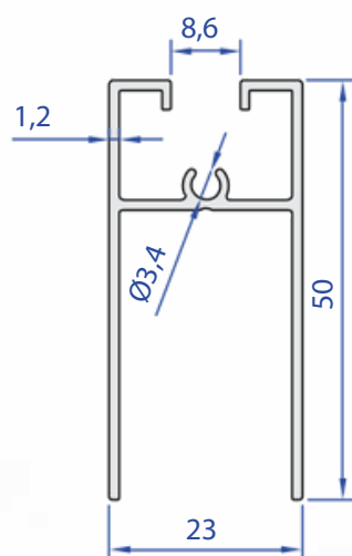
60175-00 0,466 kg/m
