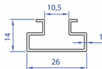
60451-00 0,192 Kg/m
