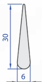
60015-00 0,292 kg/m
