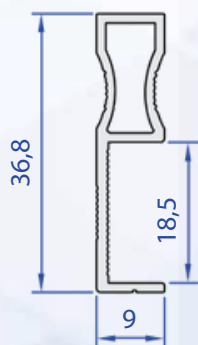
60365-00 0,269 Kg/m
