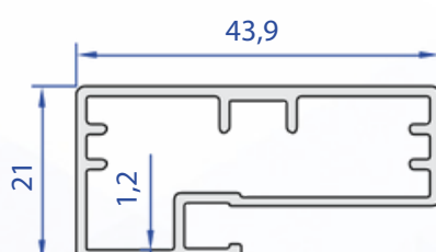
60274-00 0,506 Kg/m
