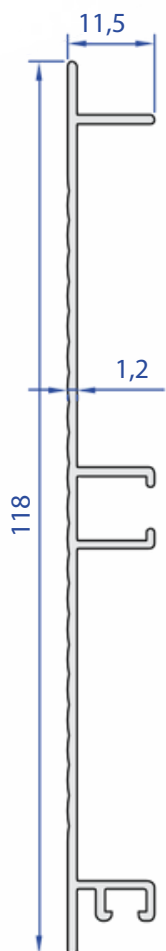
60357-00 0,527 Kg/m
