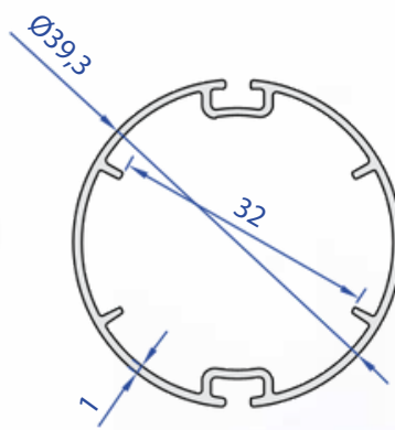
60437-00 0,405 Kg/m
