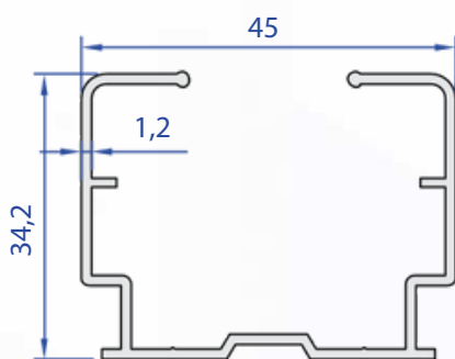
05040-00 0,473 kg/m
