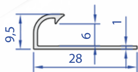
60071-00 0,116 kg/m
