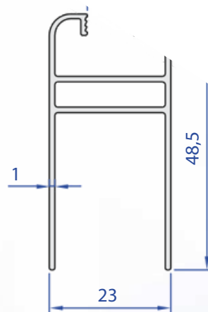
60441-00 0,417 Kg/m
