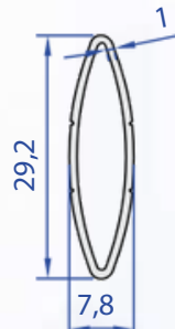
60001-00 0,161 kg/m
