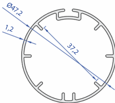
60424-00 0,594 Kg/m
