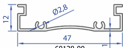
60128-00 0,260 kg/m
