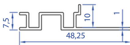
60036-00 0,224 kg/m
