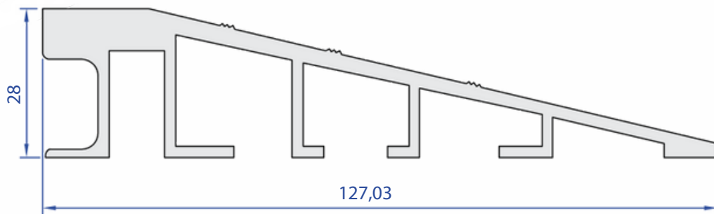
05013-00 2,045 kg/m
