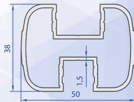
60043-00 0,910 kg/m
