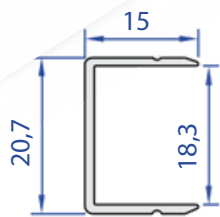
60210-00 0,151 Kg/m
