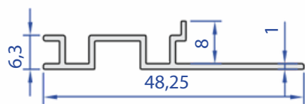
60073-00 0,209 kg/m
