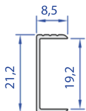
60429-00 0,095 Kg/m 19,4
