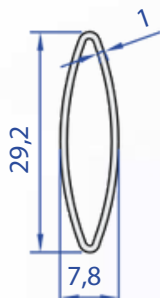
60026-00 0,162 kg/m
