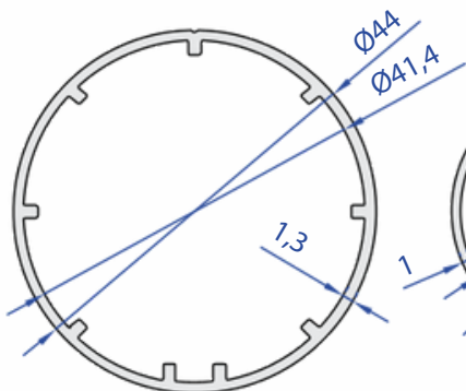
60091-00 0,538 kg/m
