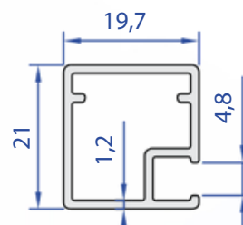
60276-00 0,286 Kg/m
