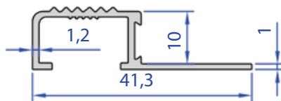
60085-00 0,223 kg/m
