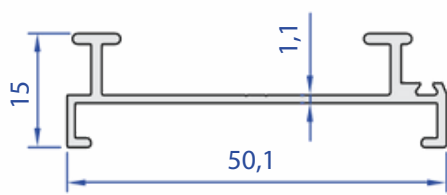
60425-00 0,308 Kg/m
