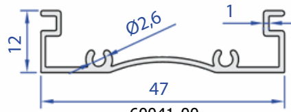
60041-00 0,266 kg/m
