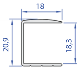
60430-00 0,159 Kg/m
