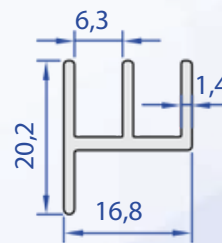
60135-00 0,222 kg/m
