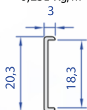
60445-00 0,064 Kg/m
