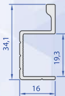
60389-00 0,284 Kg/m
