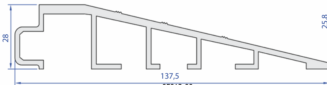
05012-00 1,835 kg/m
