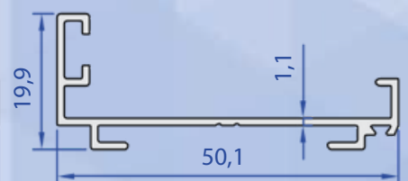
60146-00 0,306 Kg/m
