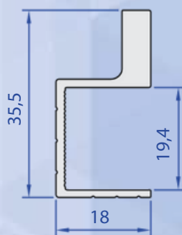
60377-00 0,430 Kg/m
