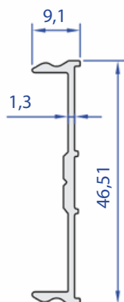
05716-00 0,251 Kg/m
