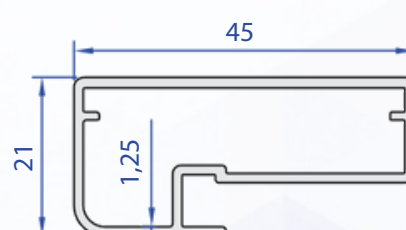
60225-00 0,476 Kg/m
