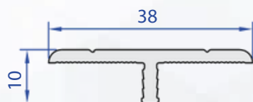
60555-00 0,294 Kg/m
