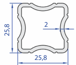
05050-00 0,506 kg/m
