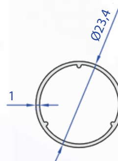
60459-00 0,280 Kg/m
