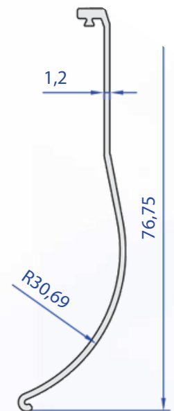
60402-00 0,307 Kg/m
