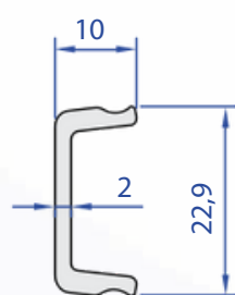
60571-00 0,210 Kg/m
