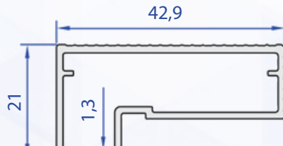
60450-00 0,477 Kg/m
