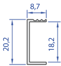
60173-00 0,091 kg/m
