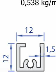
60011-00 0,174 kg/m
