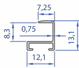
60185-00 0,074 kg/m
