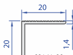
60141-00 0,135 kg/m
