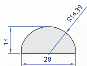
60129-00 0,847 kg/m
