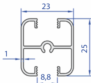
60440-00 0,292 Kg/m
