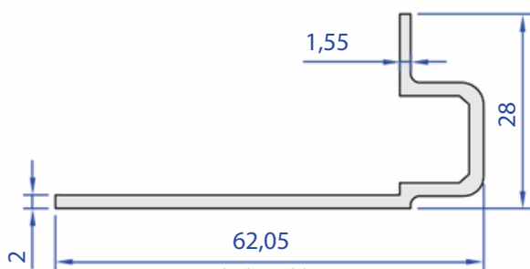
05014-00 0,513 kg/m
