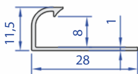
60032-00 0,121 kg/m
