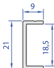
60364-00 0,138 Kg/m
