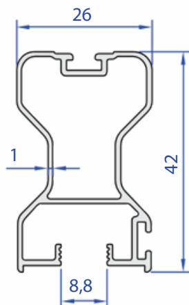
60442-00 0,455 Kg/m
