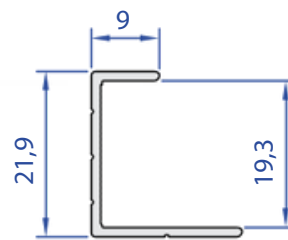
60454-00 0,168 Kg/m
