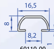
60110-00 0,086 kg/m
