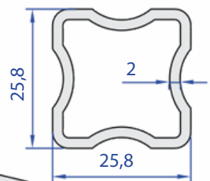
05016-00 0,515 kg/m
