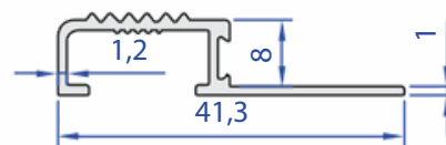
60084-00 0,210 kg/m
