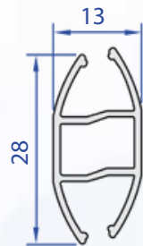
60105-00 0,226 kg/m
