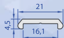
60137-00 0,130 kg/m
