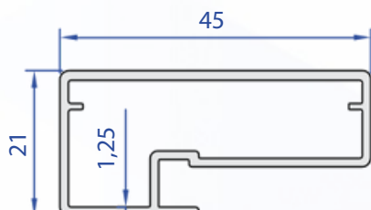
60224-00 0,480 Kg/m
