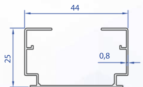
05209-00 0,275 kg/m
