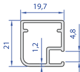
60277-00 0,282 Kg/m
