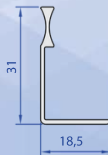
60431-00 0,170 Kg/m
