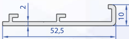
60037-00 0,382 kg/m
