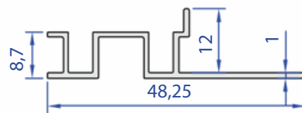
60075-00 0,239 kg/m
