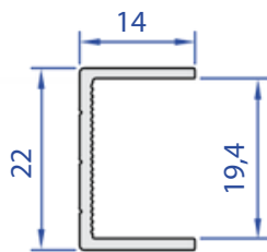
60375-00 0,176 Kg/m
