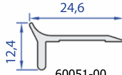
60051-00 0,129 kg/m
