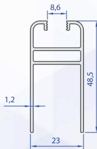
60177-00 0,496 kg/m
