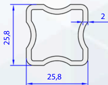
05016-00 0,515 kg/m
