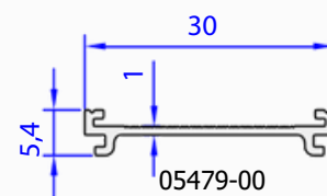
05479-00 0,113 kg/m
