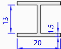
05304-00 0,215 kg/m
