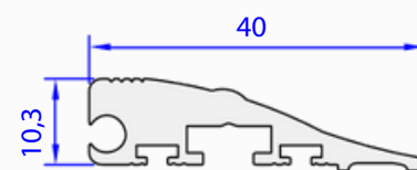
05113-00 0,503 kg/m
