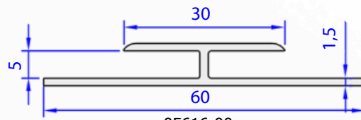
05616-00 0,382 kg/m
