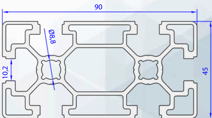
05931-00 1,390 Kg/m
