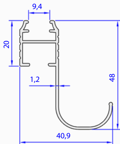
05148-00 0,395 kg/m
