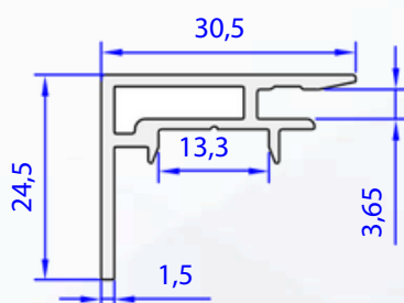
05512-00 0,331 kg/m
