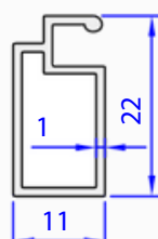
05110-00 0,179 kg/m
