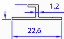
05378-00 0,104 kg/m
