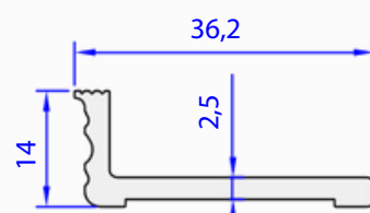
05416-00 0,339 kg/m
