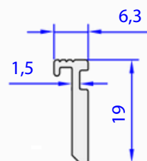
05418-00 0,154 kg/m
