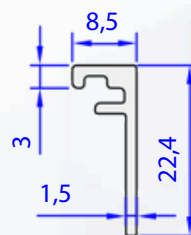
05513-00 0,152 kg/m
