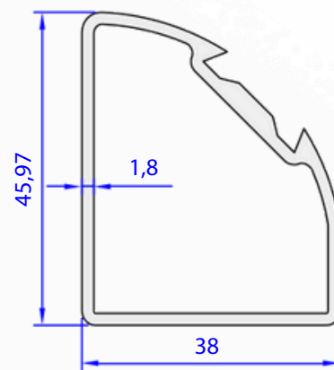
05034-00 0,782 kg/m
