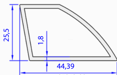
05042-00 0,555 kg/m
