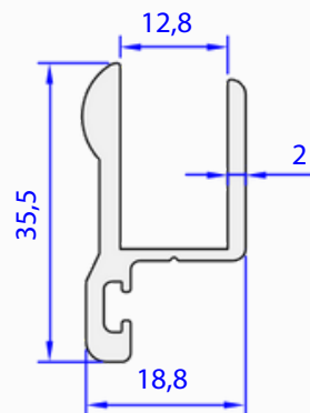
05205-00 0,477 kg/m
