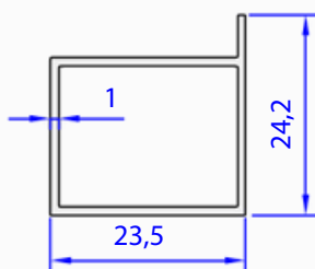
05471-00 0,234 kg/m
