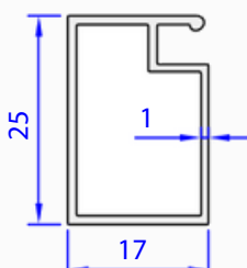
05109-00 0,234 kg/m
