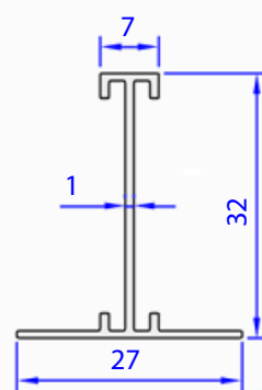
05161-00 0,195 kg/m
