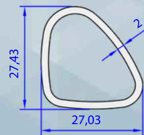
05266-00 0,446 kg/m
