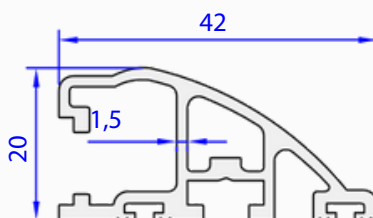
05003-00 0,575 kg/m
