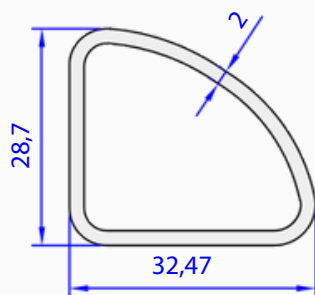
05167-00 0,528 kg/m
