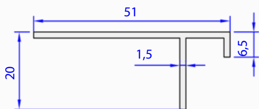
05504-00 0,303 kg/m
