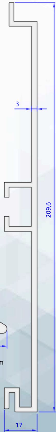
06783-00 2,244 Kg/m
