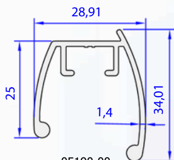
05190-00 0,411 kg/m
