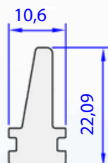
05017-00 0,357 kg/m
