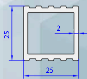
05132-00 0,545 kg/m
