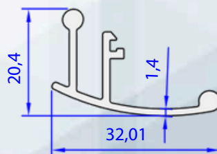
05179-00 0,290 kg/m
