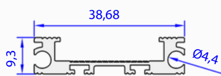
05560-00 0,322 kg/m
