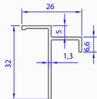
05234-00 0,221 kg/m
