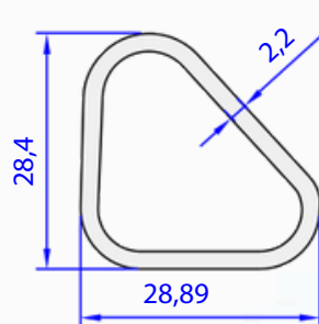
05043-00 0,515 kg/m
