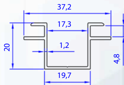
05580-00 0,278 kg/m
