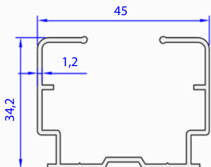
05040-00 0,473 kg/m
