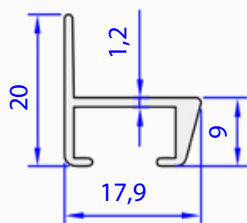
05005-00 0,142 kg/m
