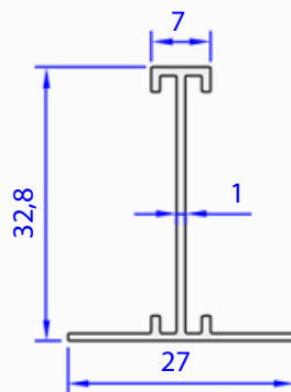
05210-00 0,197 kg/m
