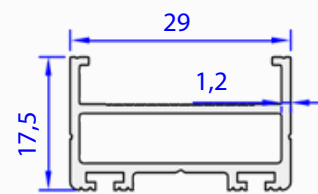
05329-00 0,324 kg/m
