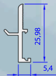
05051-00 0,164 kg/m
