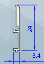
05129-00 0,108 kg/m
