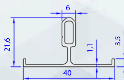
05546-00 0,260 kg/m
