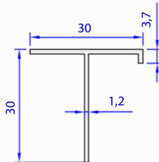
05212-00 0,199 kg/m
