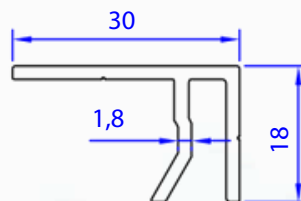
06541-00 0,309 Kg/m
