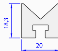
05134-00 0,664 kg/m
