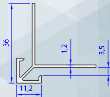
05376-00 0,291 kg/m
