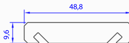
05112-00 1,168 kg/m
