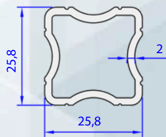
05050-00 0,506 kg/m
