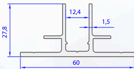
05359-00 0,717 kg/m
