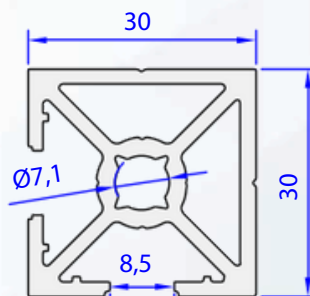
06734-00 0,884 Kg/m
