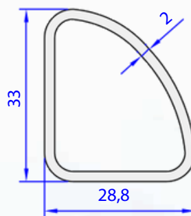
05128-00 0,533 kg/m
