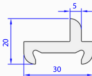
05548-00 0,608 kg/m
