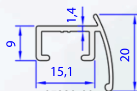
05229-00 0,194 kg/m
