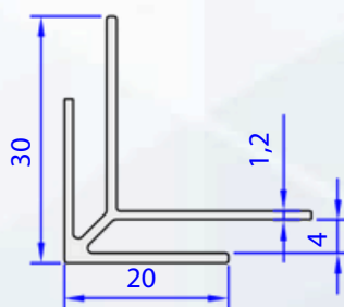
05353-00 0,304 kg/m
