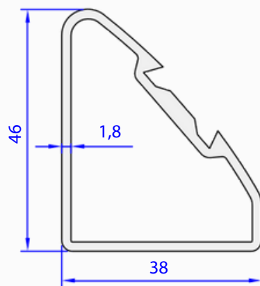
05007-00 0,768 kg/m
