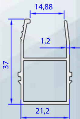
05344-00 0,381 kg/m
