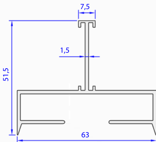
05160-00 0,725 kg/m
