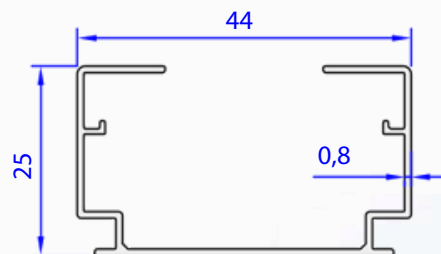
05209-00 0,275 kg/m
