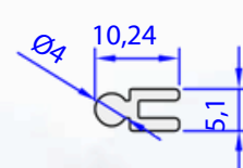
05114-00 0,090 kg/m
