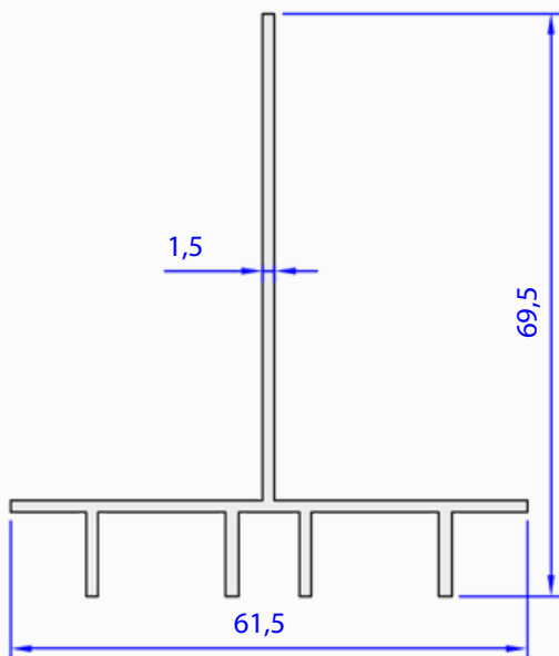
06243-00 0,648 Kg/m
