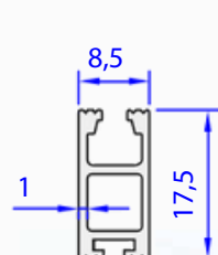
05018-00 0,230 kg/m
