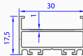
05462-00 0,288 kg/m
