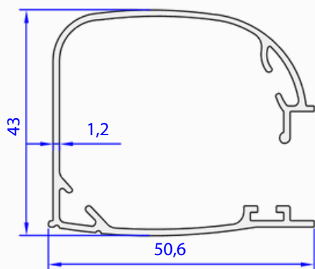
05108-00 0,594 kg/m
