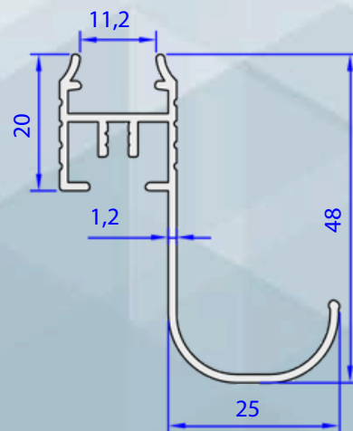
05064-00 0,423 kg/m
