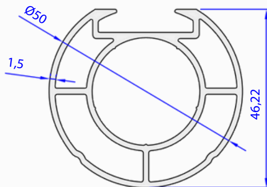
06669-00 1,141 Kg/m
