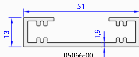
05066-00 0,545 kg/m
