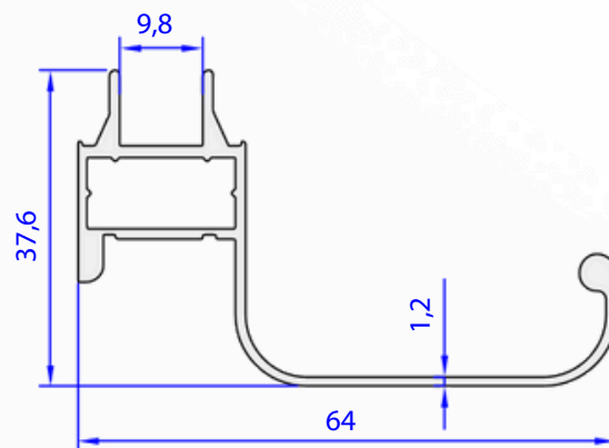
05343-00 0,564 kg/m
