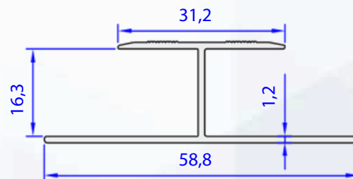
05653-00 0,346 kg/m
