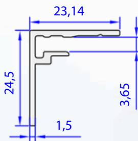
05514-00 0,224 kg/m
