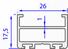
05002-00 0,309 kg/m
