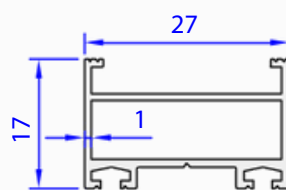
05157-00 0,269 kg/m
