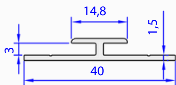
05617-00 0,233 kg/m
