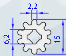
05567-00 0,301 kg/m
