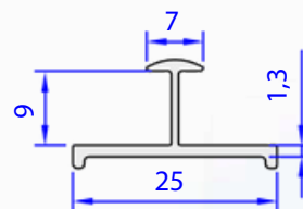
05430-00 0,147 kg/m
