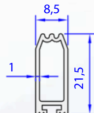
05037-00 0,166 kg/m
