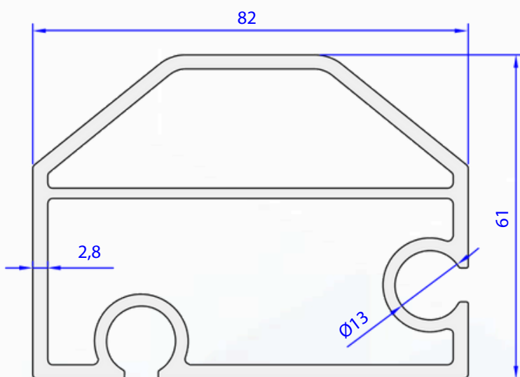
07013-00 2,613 Kg/m
