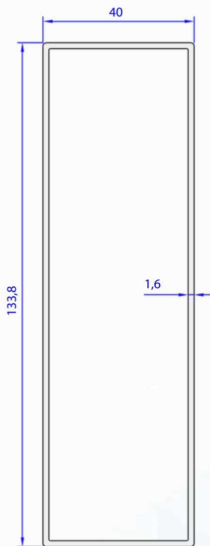
07016-00 1,477 Kg/m
