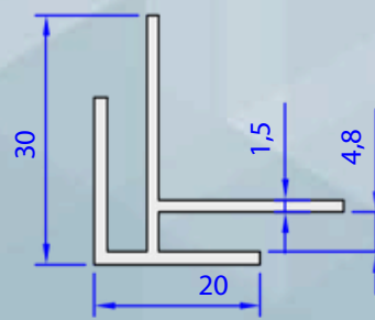
05058-00 0,363 kg/m
