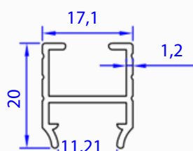
05073-00 0,205 kg/m
