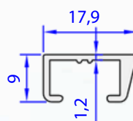
05057-00 0,142 kg/m
