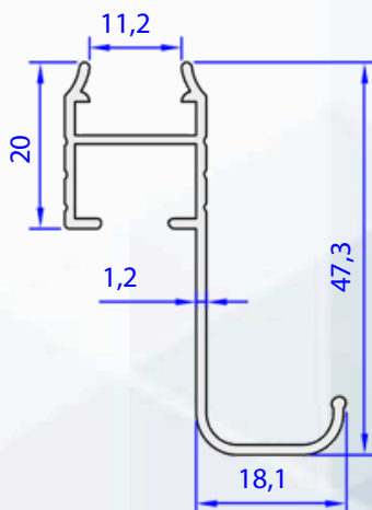
05072-00 0,356 kg/m
