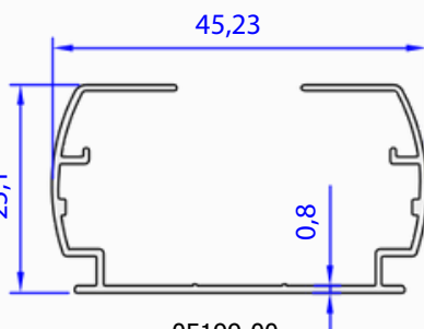
05199-00 0,288 kg/m
