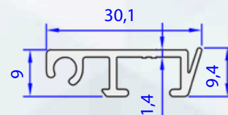
05178-00 0,246 kg/m
