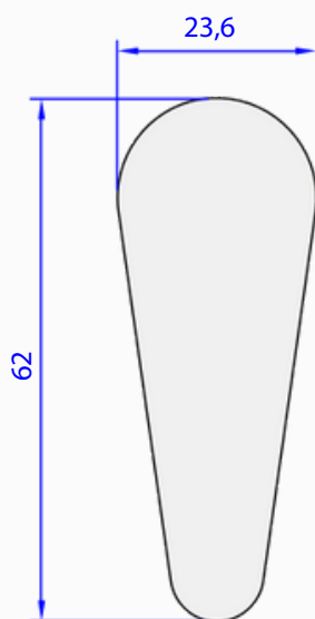
05094-00 2,839 kg/m
