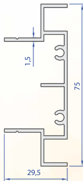
45005-00 0,768 kg/m
