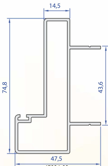
45004-00 0,982 kg/m
