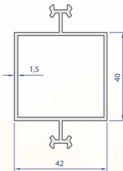
45003-00 0,853 kg/m
