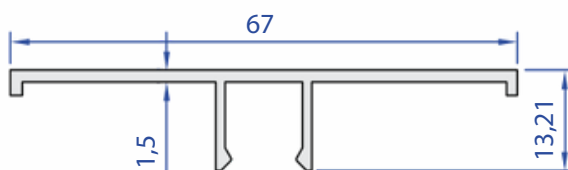
45006-00 0,369 kg/m
