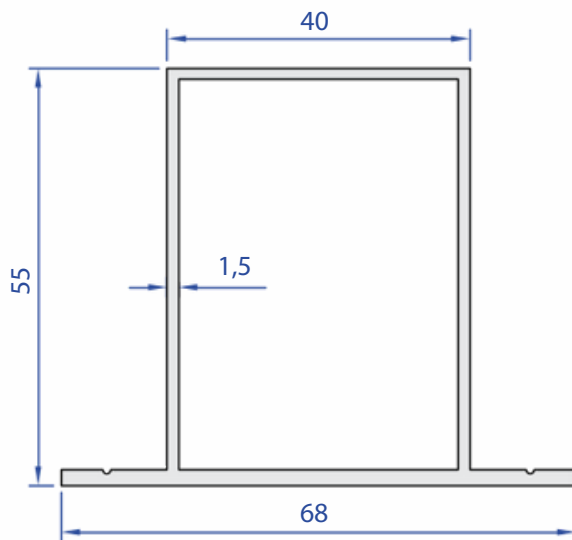
45001-00 0,948 kg/m
